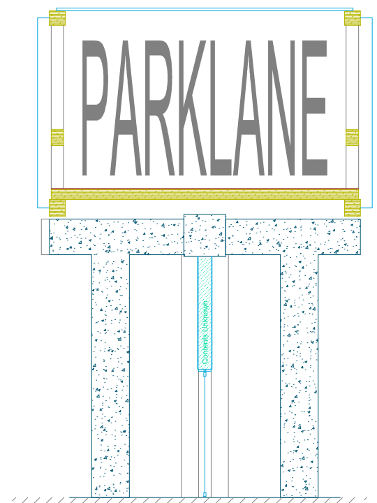
Section A-A 1/100
